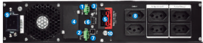
Painel traseiro do no-break modelo 9PX3000IB
